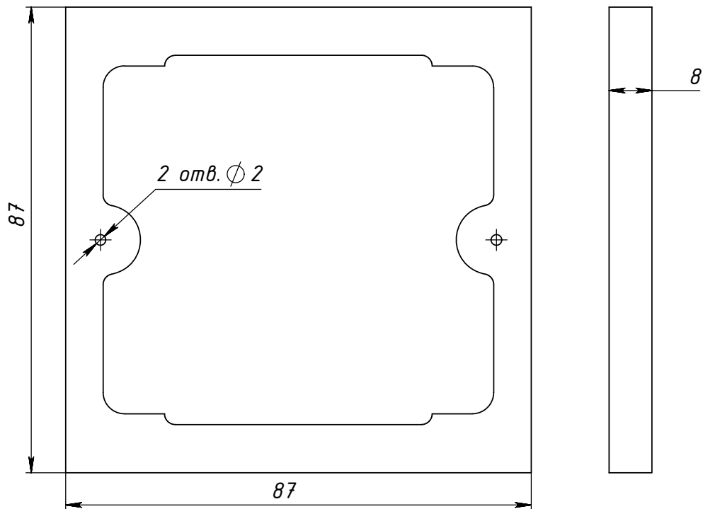
Деталь 2_МДФ 8 мм
