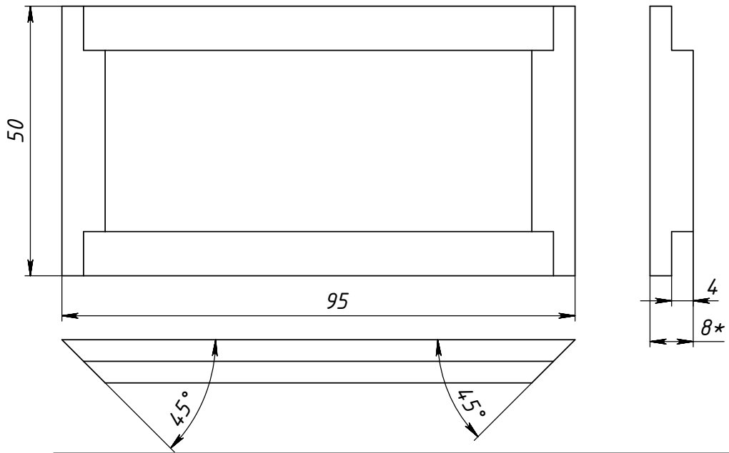
Деталь 2_МДФ 8 мм
