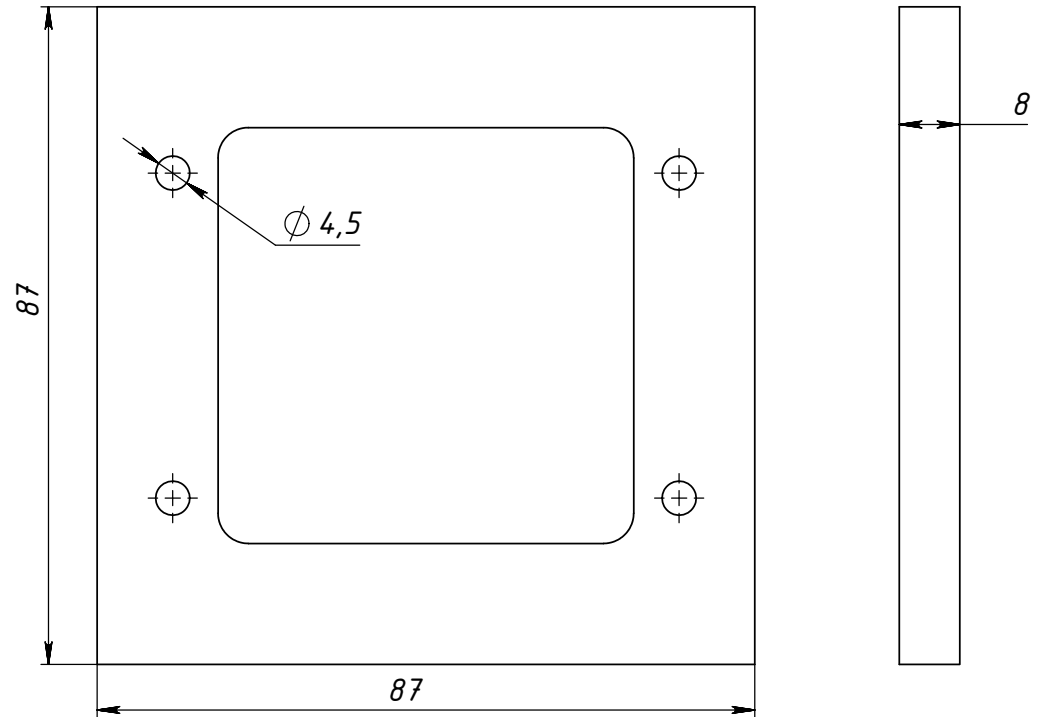
Деталь 3_МДФ 8 мм
